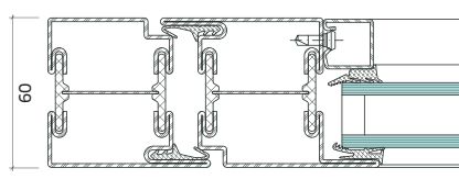
Porta in acciaio Janisol profilo (isolato)
