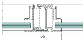
Jansen Art'15 profilo
