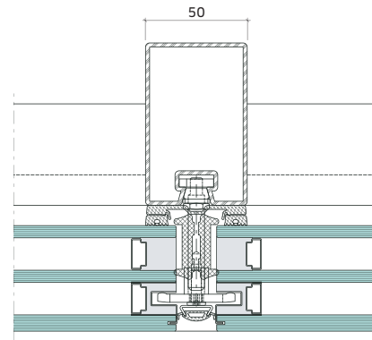
Facciata VISS SG profilo
