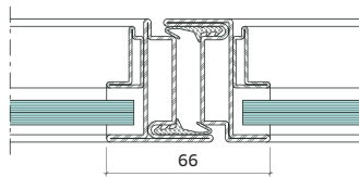
Profilé Jansen Art'15
