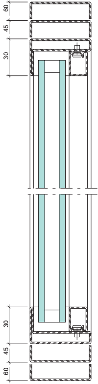
E - E
