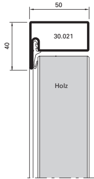
B - B
