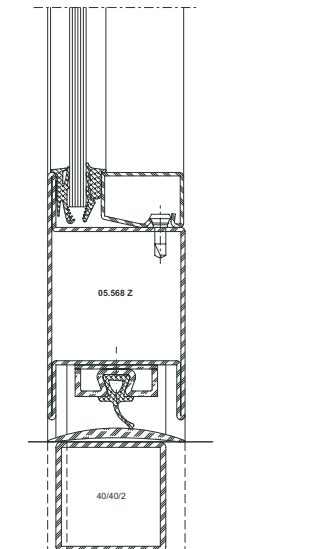
Barrier-free door
