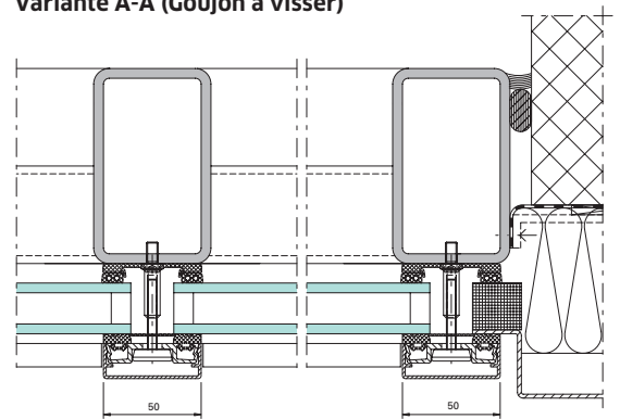
Variante A-A (Goujon à visser)
