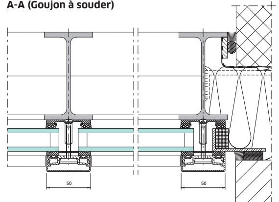
A-A (Goujon à souder)
